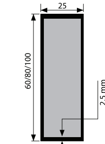
Przekrój podłużnicy Sides with reinforced section Řez podélníci 2,5 mm
